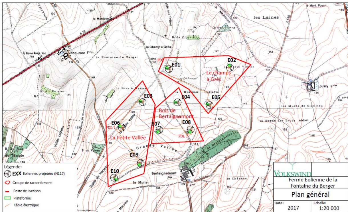
Carte 6 : Carte de localisation du réseau inter-éolienne
