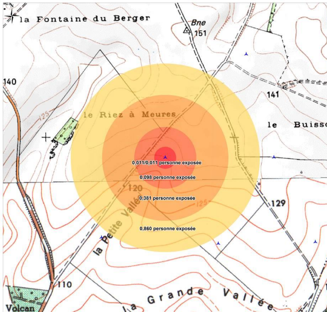
Carte 10 : Synthèse des risques de l'éolienne E03
