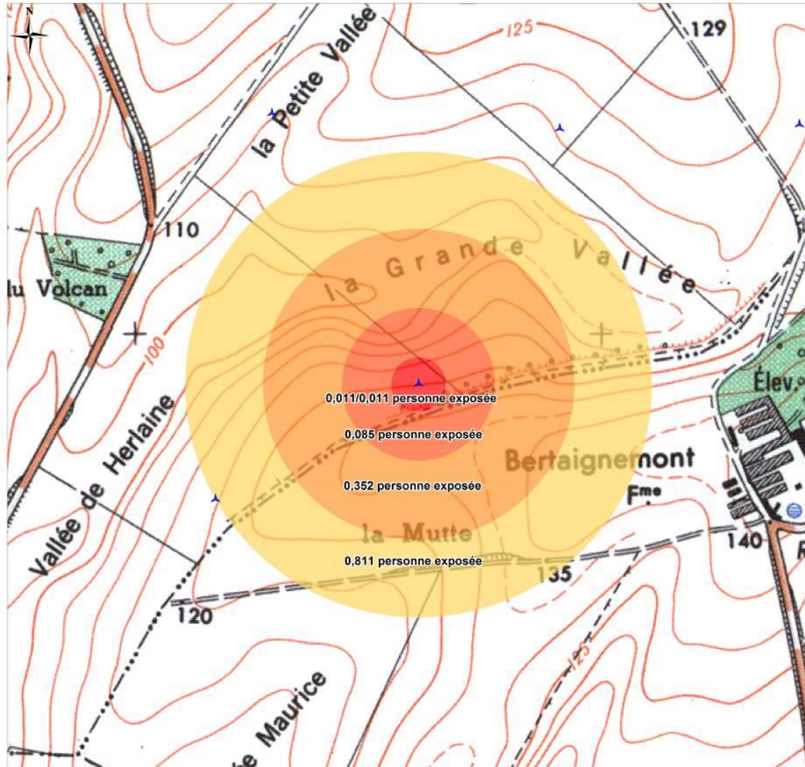
Carte 16 : Synthèse des risques de l'éolienne E09
