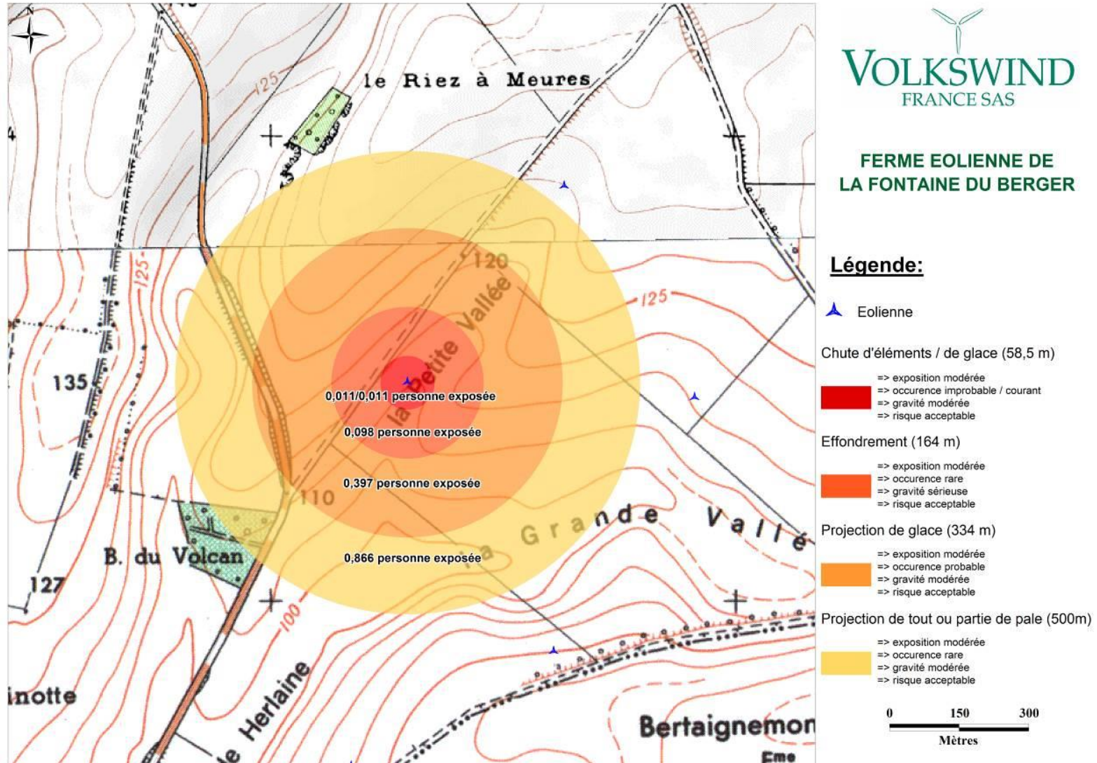
Carte 13 : Synthèse des risques de l'éolienne E06
