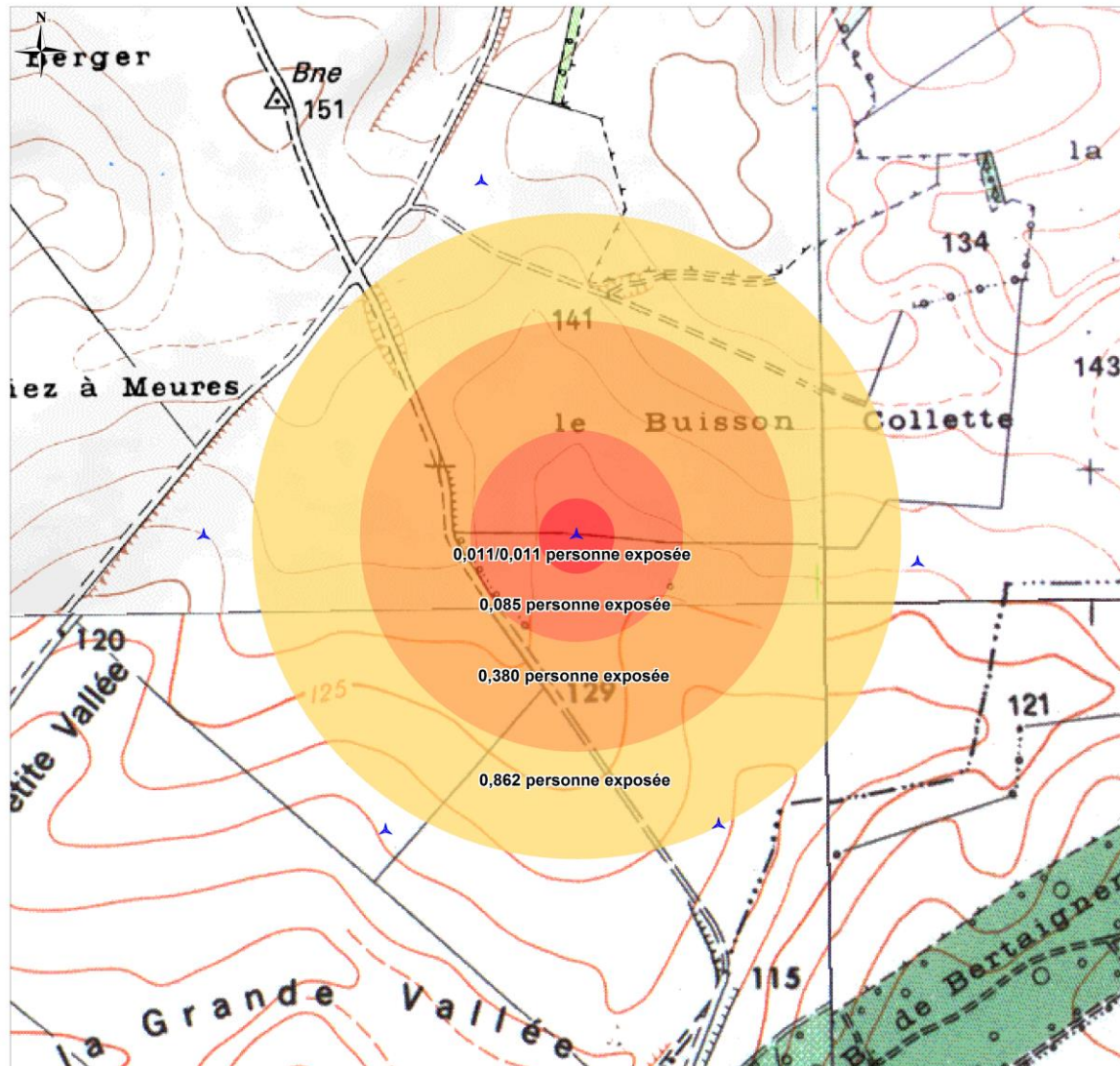
Carte 11 : Synthèse des risques de l'éolienne E04
