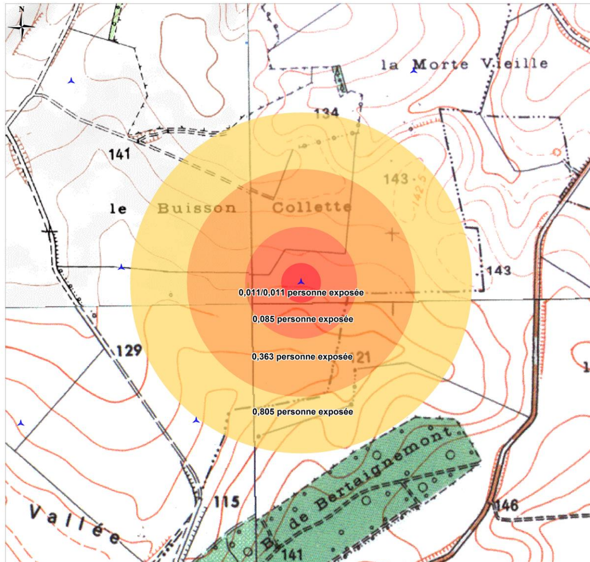
Carte 12 : Synthèse des risques de l'éolienne E05
