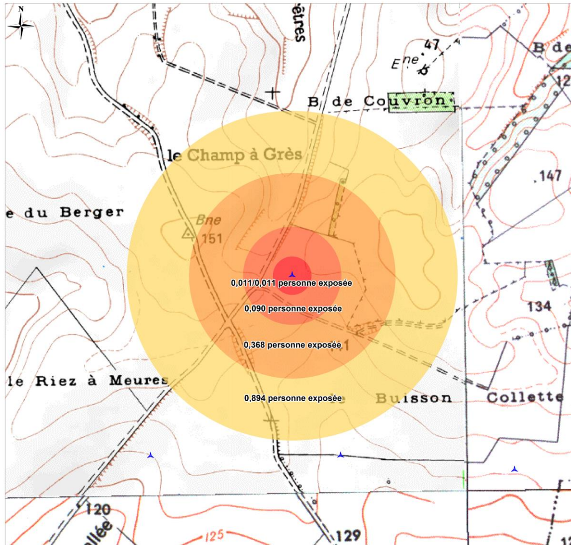
Carte 8 : Synthèse des risques de l'éolienne E01
