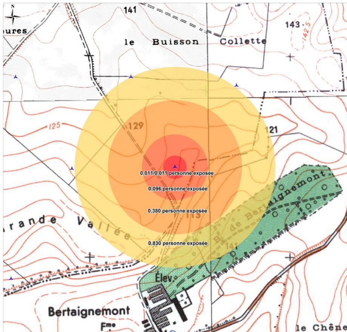
Carte 15 : Synthèse des risques de l'éolienne E08
