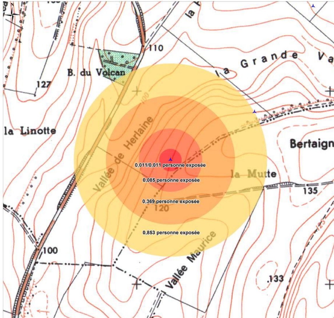
Carte 17 : Synthèse des risques de l'éolienne E10
