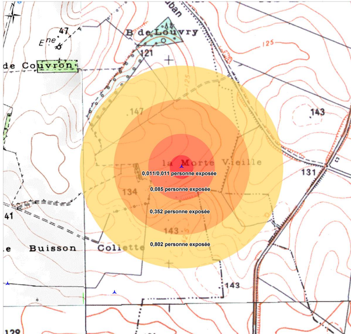
Carte 9 : Synthèse des risques de l'éolienne E02
