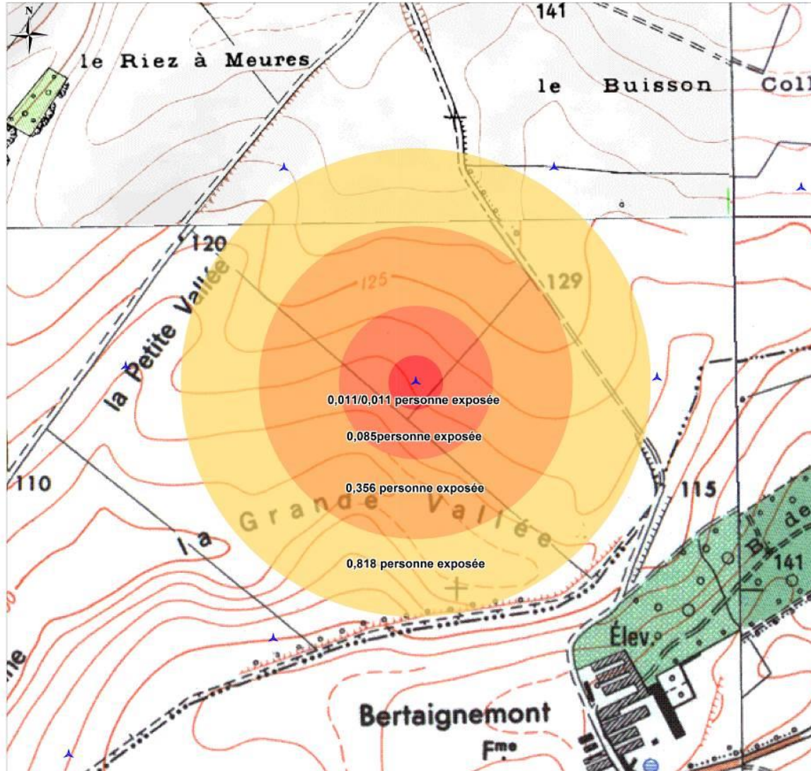
Carte 14 : Synthèse des risques de l'éolienne E07
